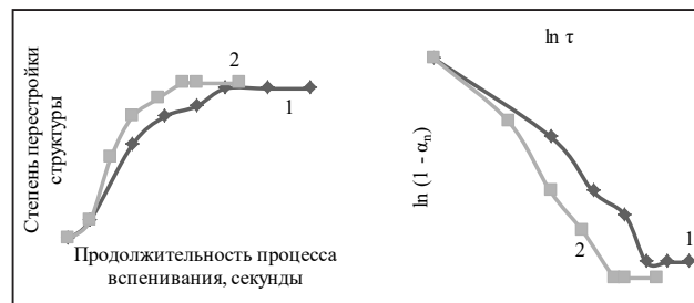
Рис. 5. Зависимости: а) степени перестройки структуры от продолжительности процесса вспенивания с использованием алюминиевой пудры; б) \ln(1-\alpha_n) = f(\ln \tau) при разных температурах (1 – при +10°C; 2 – при +20°C)
