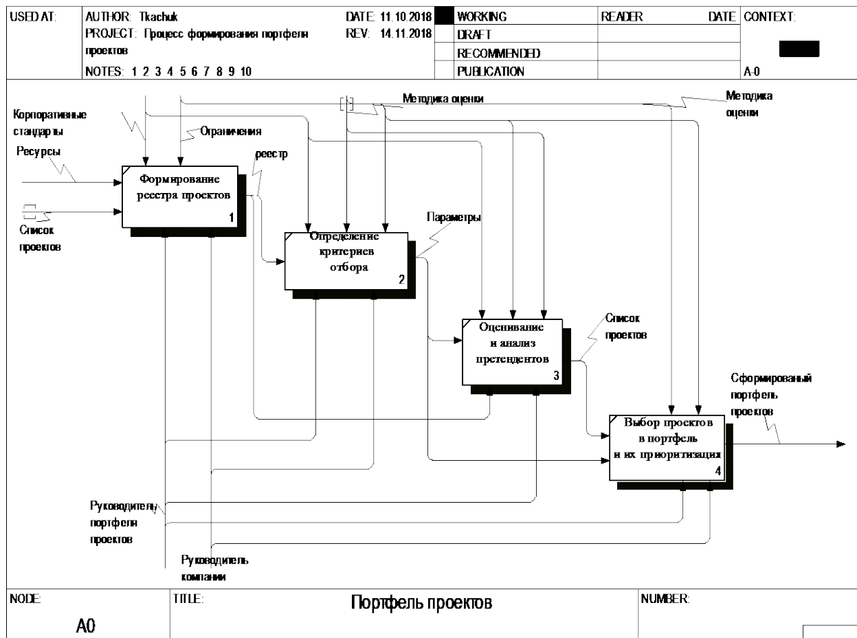
Рис. 2. Модель процесу формування портфелю проектів
