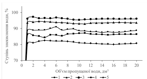
Рис. 6. Залежність ступеню знекиснення води від об'єму пропущеної водопровідної (1; 2) та Na + -катіонованої (3; 4; 5) води через редоксит МЗ та катіоніт КУ-2-8 в Na + -формі (2; 3; 4; 5) при швидкостях фільтрування, м/год: 2,12 (1; 2; 3); 6,36 (4); 10,6 (5); рН: 7,500 (1; 2); 7,851 (3; 4; 5); [O 2 ], мг/дм 3 : 8,05 (1); 9,23 (2); 9,74 (3; 4; 5)
