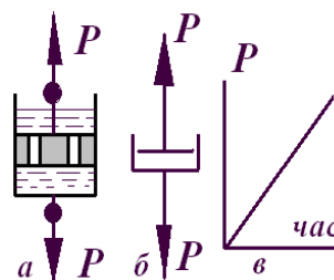
Рис. 5. Модель-імітатор в'язкого тіла (реологічне тіло Ньютона)
