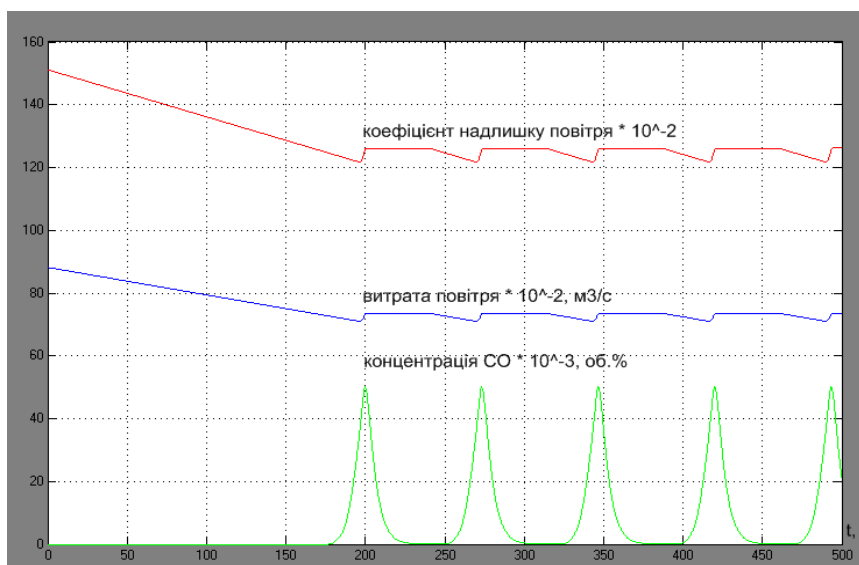
Рис. 7. Результати моделювання при G_{\text{палива}} = 120 \text{ м}^3/\text{год} і G_{\text{пов}} = 12,6 \cdot G_{\text{палива}}
