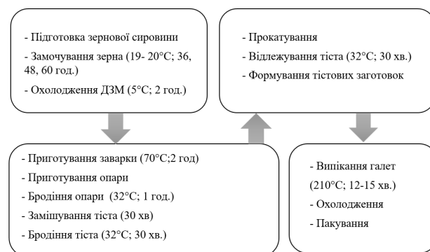
Рис. 2. Функціонально-параметрична схема виробництва галет із диспергованою кукурудзою
