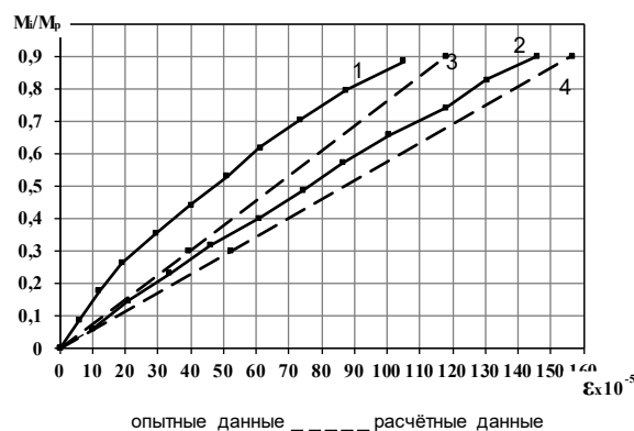
Рис. 1. Зависимость средних деформаций сжатой грани бетона \varepsilon_{sc}^{exp} от изгибающего момента при различном армировании
