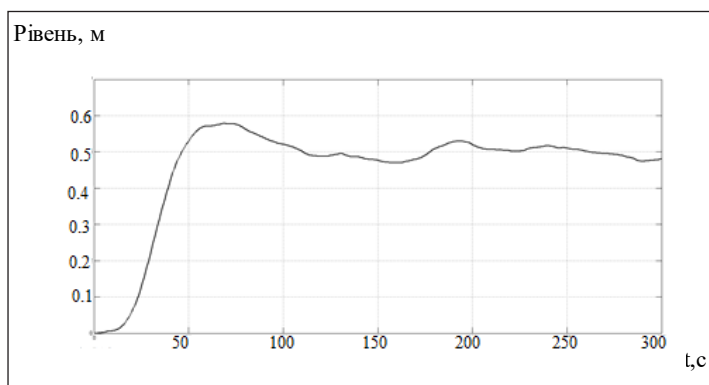
Рис. 2. Перехідний процес зміни рівня у змішувачі
