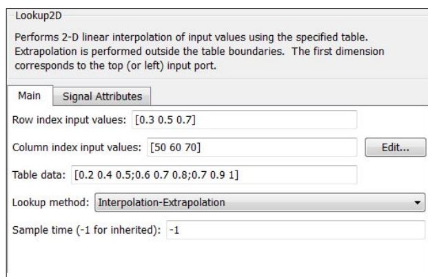
Рис. 11. Блок Lookup2D Table
