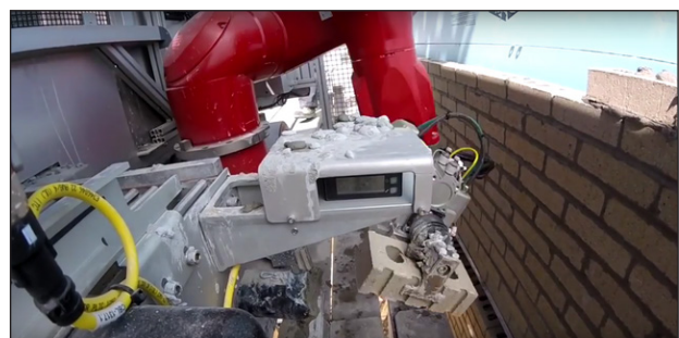
Рис. 2. Напіваавтоматичний робот SAM компанії Construction Robotics [10]
