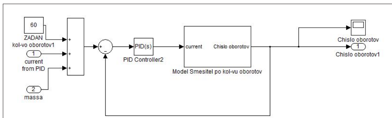
Рис. 8. Структура підсистеми Stabilizacia Cisl oborotov
