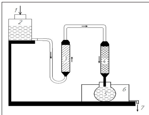
Рис. 1. Експериментальна установка для знекиснення води
