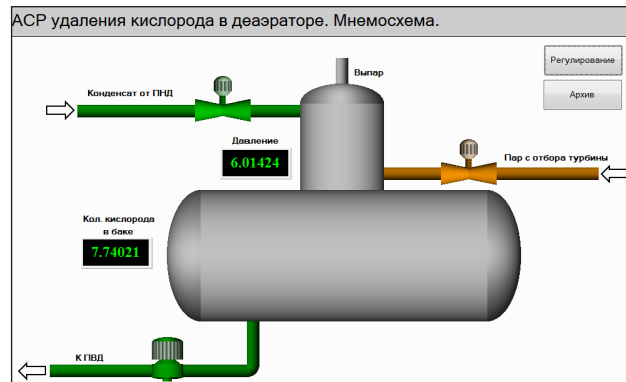
Рис. 3. Мнемосхема объекта автоматизации
