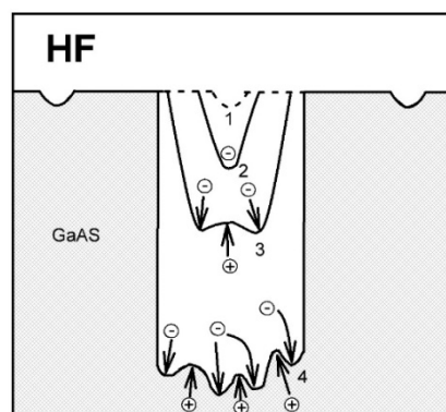
Рис. 2. Схематична ілюстрація механізму формування \text{por-GaAs}
