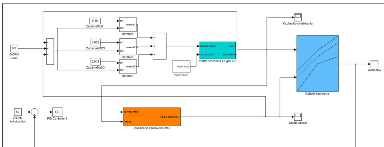
Рис. 3. Модель управління якістю змішування продукції
