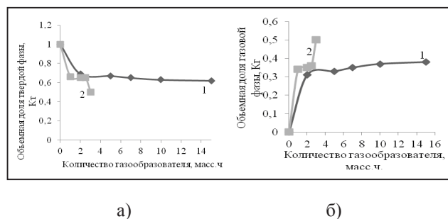
Рис. 2. Влияние газообразующего агента на объемную долю твердой (а) и газовой (б) фаз пеноматериала (1 – перекись водорода; 2 – алюминиевая пудра)
