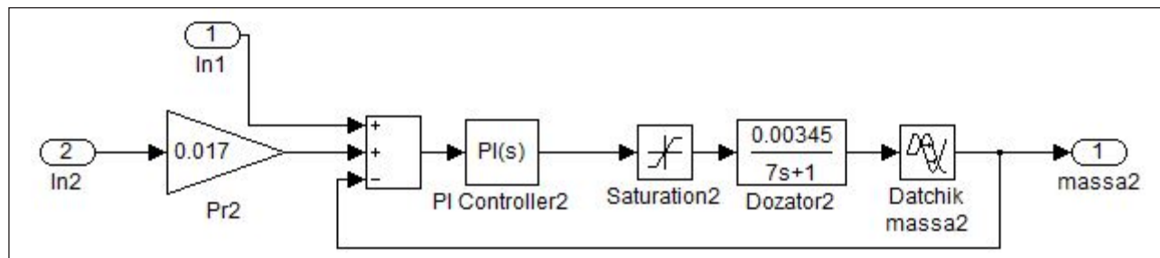
Рис. 5. Структура підсистеми Massa2
