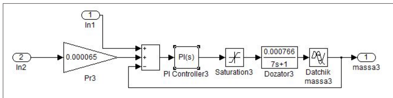
Рис. 6. Структура підсистеми Massa3
