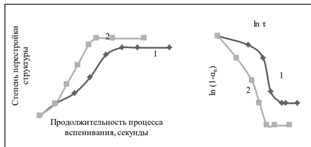
Рис. 4. Зависимости: а) степени перестройки структуры от продолжительности процесса вспенивания с использованием перекиси водорода; б) \ln(1-\alpha_n) = f(\ln \tau) при разных температурах (1 – при +10°C; 2 – при +20°C)
