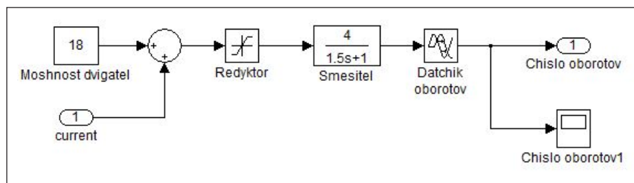
Рис. 9. Структура підсистеми Model Smesitel po kol-vu oborotov
