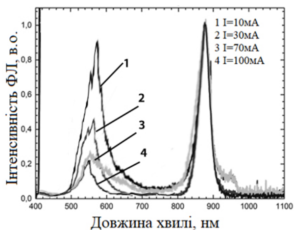
Рис. 6. Фотолюмінесценція зразків porousGaAs, отриманих за струмів травлення 10 \div 100 \text{ mA}
