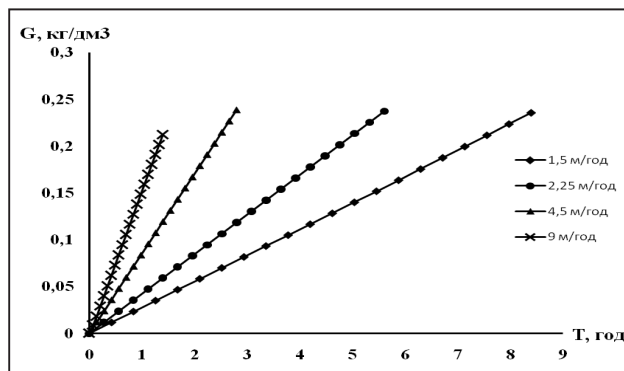
Рис. 1. Залежність питомої брудомісткості фільтру від часу фільтрування при різних швидкостях фільтрування води
