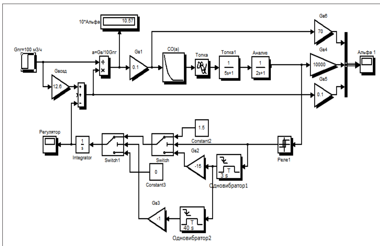
Рис. 4. Схема моделювання АСР економічності спалювання палива
