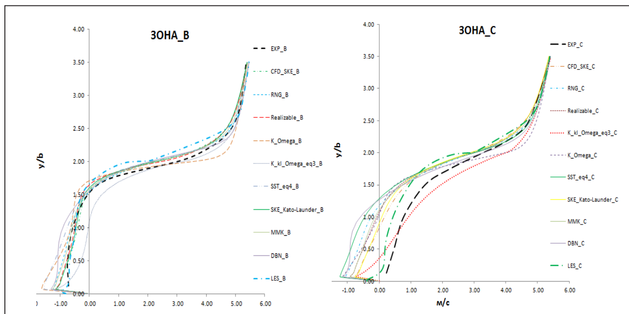
Рис. 4. Вертикальное распределение скорости ветра над зданием
