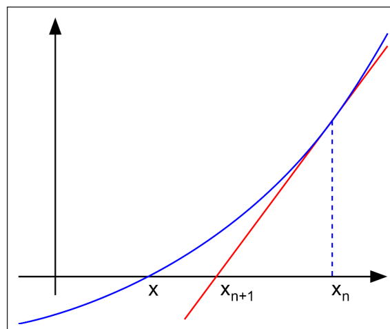
Рис. 1. Иллюстрация метода Ньютона
