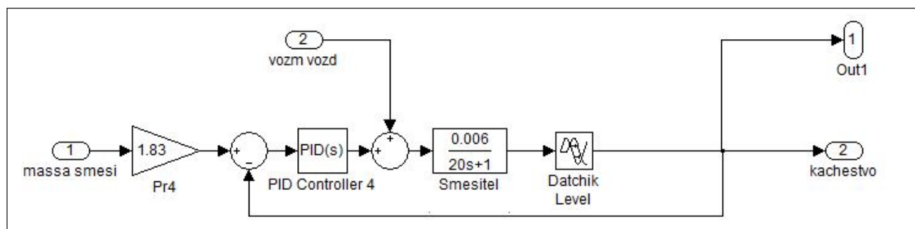
Рис. 7. Структура підсистеми Model smesitela po urovny
