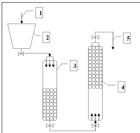
Рис. 1. Двостадійна схема знезалізнювання води 1 – вихідна вода; 2 – резервуар подачі води; 3 – фільтр із магнітним сорбентом; 4 – фільтр із завантаженням сополімеру стиролу та дивінілбензолу; 5 – очищена вода.
