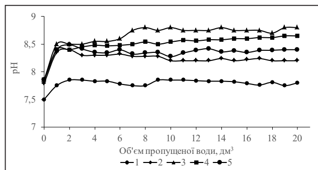
Рис. 4. Залежність рН від об'єму пропущеної водопровідної (1, 2) та \text{Na}^+ -катіонованої води (3; 4; 5) через редоксит МЗ (1) та катіоніт КУ-2-8 в \text{Na}^+ -формі (2; 3; 4; 5) при різних швидкостях фільтрування, м/год: 2,12 (1; 2; 3); 6,36 (4); 10,6 (5)
