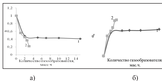
Рис. 3. Влияние газообразующего агента на: а) параметр структурообразования; б) степень перестройки структуры пеноматериала (1 – перекись водорода; 2 – алюминиевая пудра)
