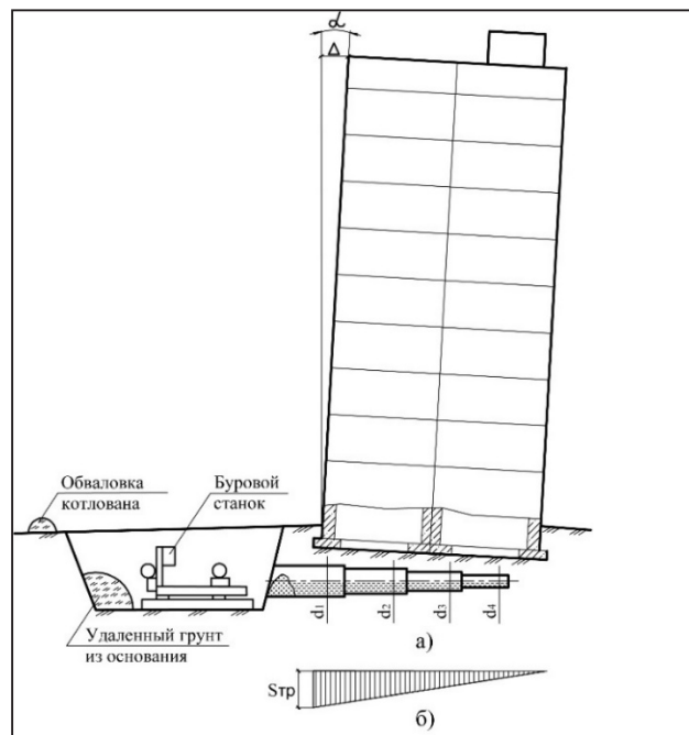
Рис. 2. Технологічна схема вирівнювання будівлі в поперечному напрямі: а) параметри поперечного крену і свердловини змінного перетину; б) епіюра необхідних технологічних осідань фундаментів
