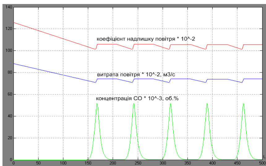
Рис.5. Результати моделювання при G_{\text{палива}} = 100 \text{ м}^3/\text{год} і G_{\text{пов}} = 12,6 \cdot G_{\text{палива}}
